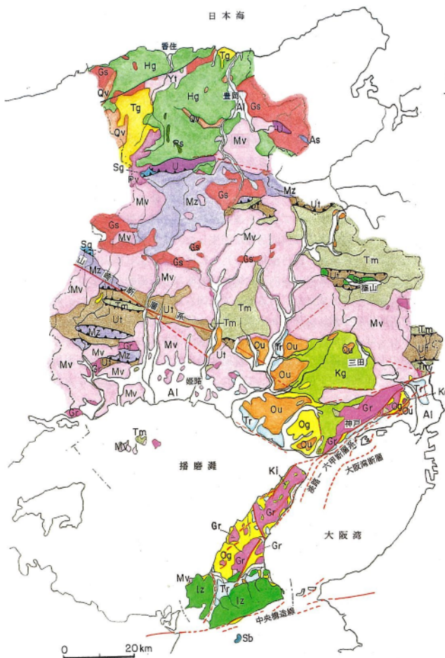
----- 地帯境界断層 ———— 主な活断層 (確実度 I) - - - - - 主な活断層 (伏在部, 確実度 II)
