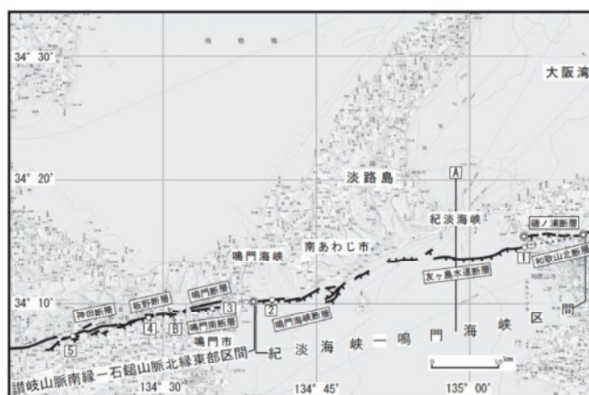
図2-2 中央構造線断層帯の活断層位置と主な調査地点 1：紀淡海峡地点 2：鳴門海峡地点 3：段間・大代地点 4：川端A、B地点 5：熊谷寺東南地点 A：文献39 B：文献34 活断層の位置は文献4、11、14、17、22に基づく。 .....：活断層が地表に現れていない区間 ◎：活動区間の奥端および境界 ⊕：紀淡海峡-鳴門海峡の活動区間のうち、第四紀後期における活動性が確かめられている区間の東端 基図は国土院発行数値地図200000「和歌山」及び「徳島」を使用。
